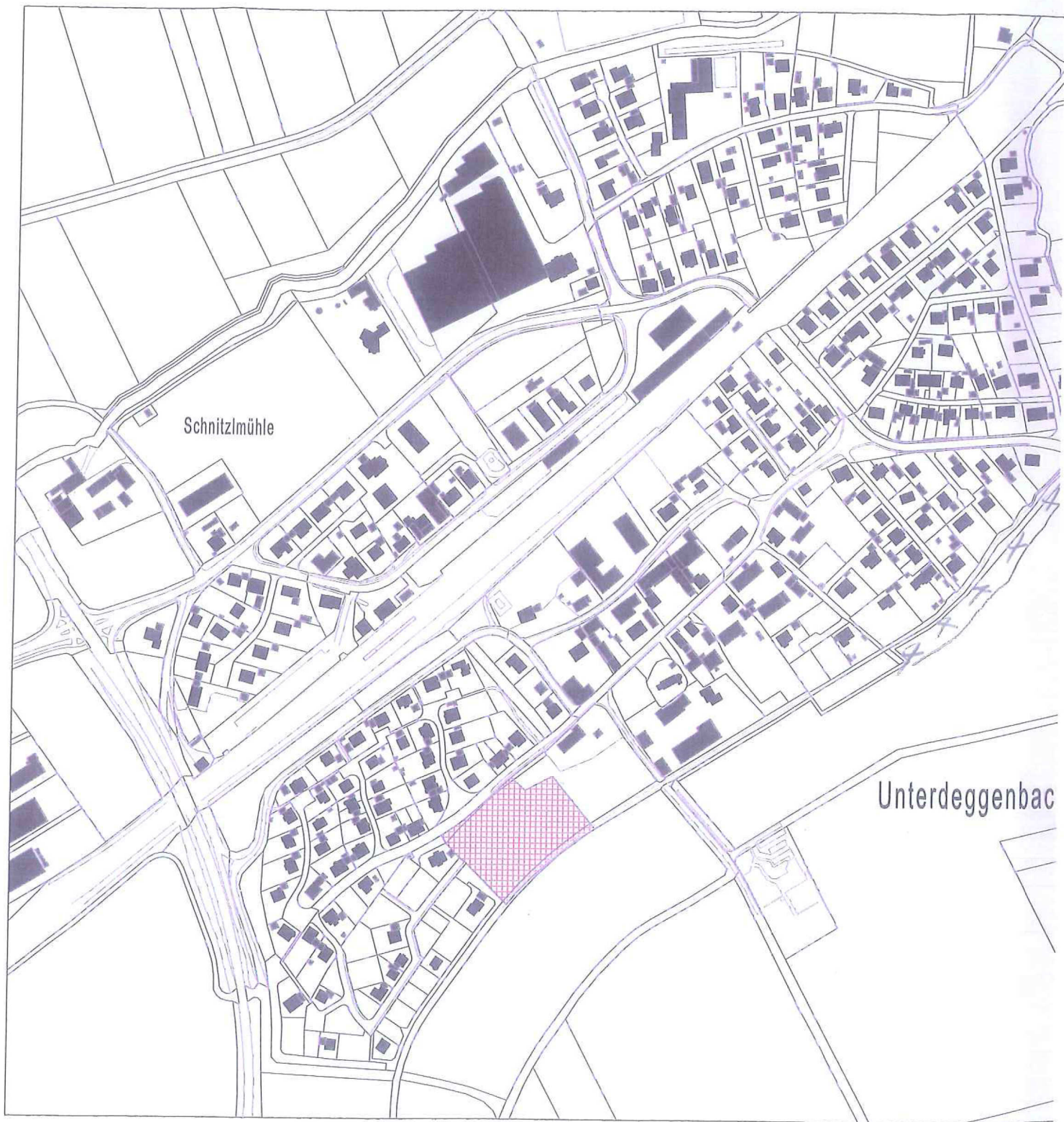
Übersichtslageplan M=1/5000
