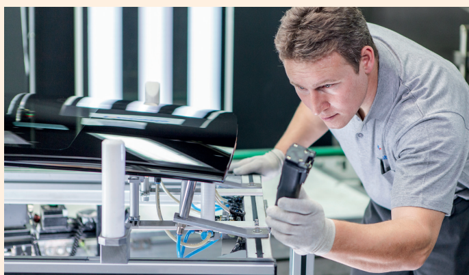
In Schierling wird das weltweit größte Panoramadach aus Polycarbonat gebaut.
